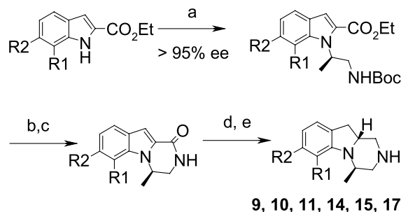
Scheme 2. Reagents and conditions: (a) NaH, DMF, then ( S )- 3 ; (b) TFA, CH 2 Cl 2 ; (c) MeOH, K 2 CO 3 ; (d) LiAlH 4 , Et 2 O, reflux; (e) NaBH 4 , TFA, THF.
